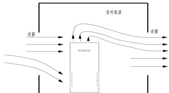
图 6 室外机房水平自然对流示意图
