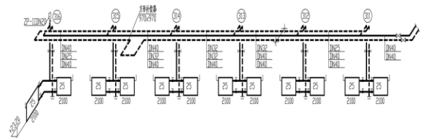
图5 室外机房间供暖系统图
