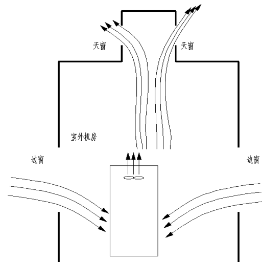
图 7 室外机房垂直气流示意图
