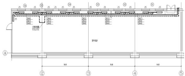
图4 室外机房供暖平面图
