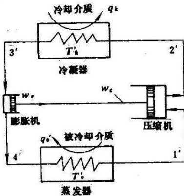
图2 卡诺循环
