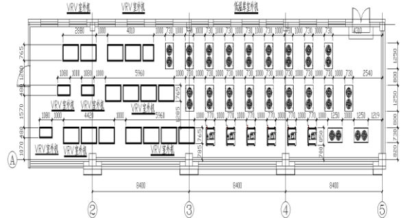
图3 直膨式空调室外布置图
