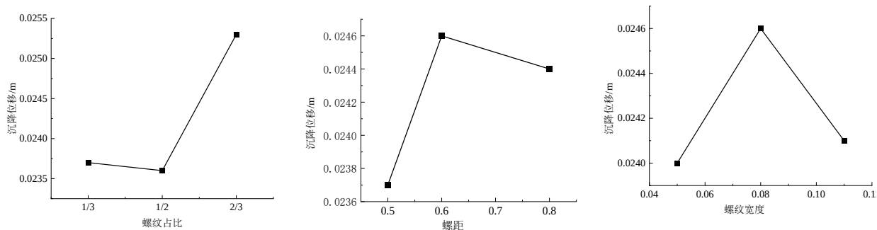
图6 螺紋桩沉降位移随螺紋占比的变化曲线
