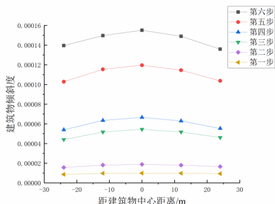
图6 各开挖步骤建筑物倾斜度图
