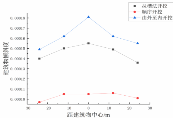
图 11 不同开挖顺序对应的建筑物倾斜度
