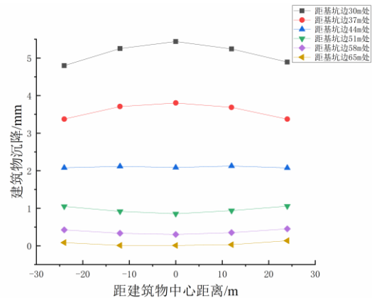
图5 建筑物沉降量图
