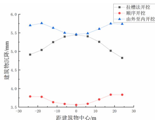
图9 不同开挖顺序对建筑物沉降的影响
