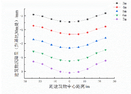
图3 不同钢支撑水平间距建筑物沉降量
