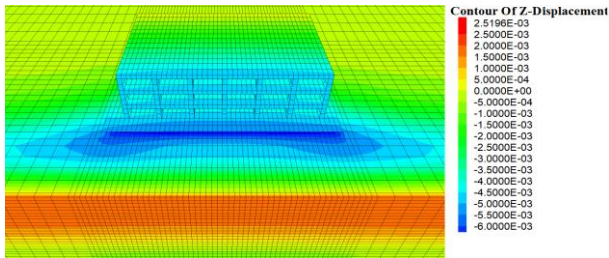
(c) 由外至内开挖
