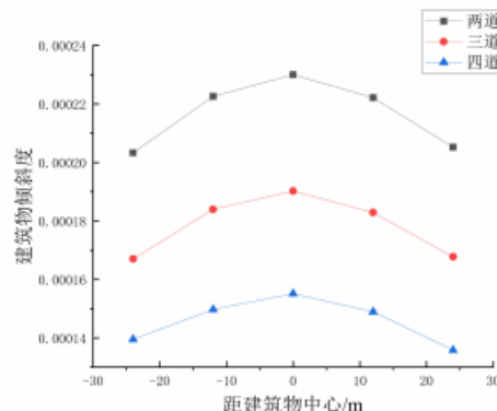
图8 不同钢支撑道数对应建筑物倾斜度
