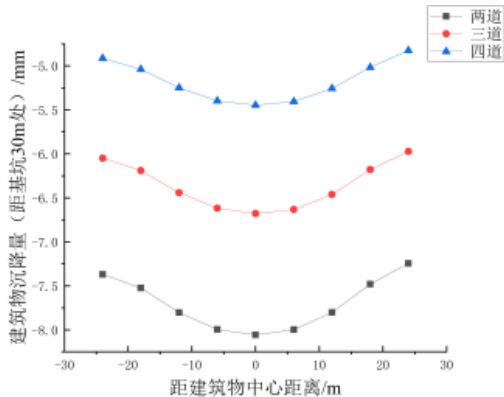
图4 不同钢支撑道数对应的建筑物沉降量曲线图
