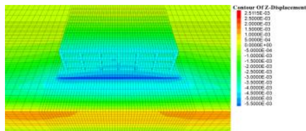
(a) 拉槽法开挖
