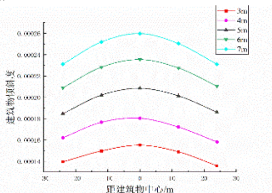
图7 各钢支撑间距建筑物倾斜度图
