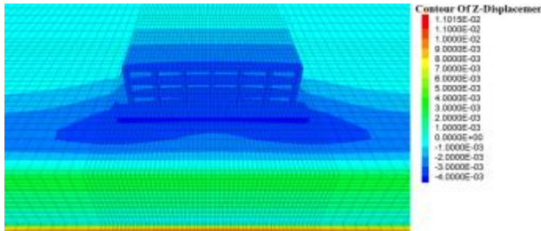
(b) 顺序开挖
