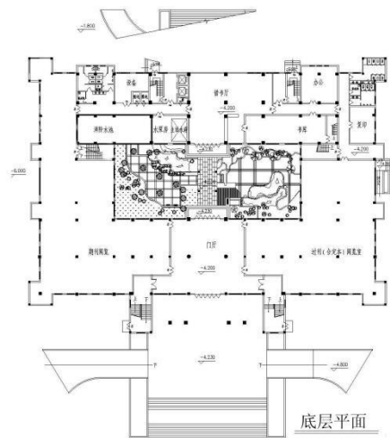
图3 底层平面
