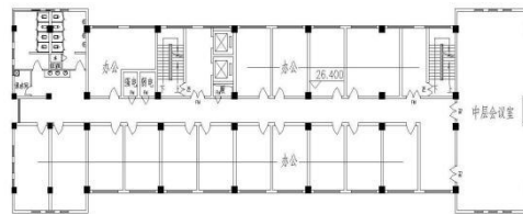
图4 标准层平面
