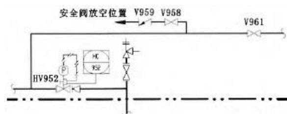
图 1 再生气体的装置入口增加排气阀
