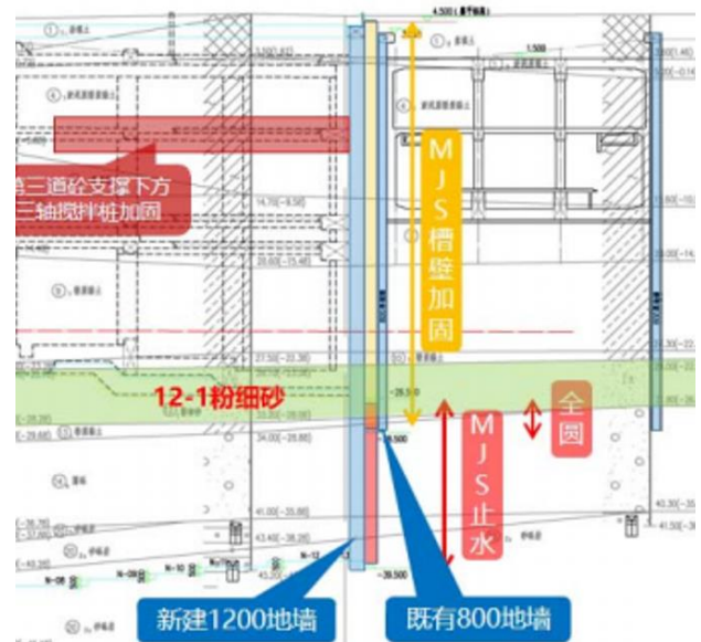
图5 某车站地保区 MJS 加固剖面图
