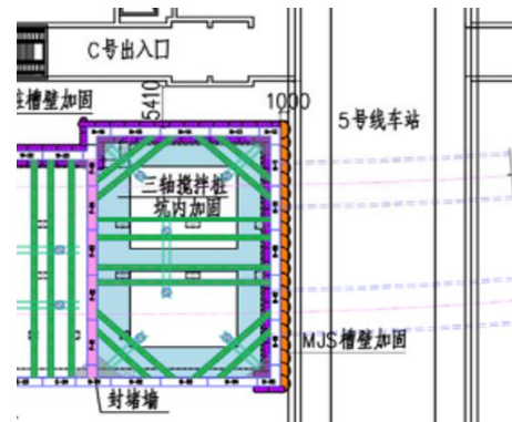
图4 某车站地保区 MJS 加固平面图
