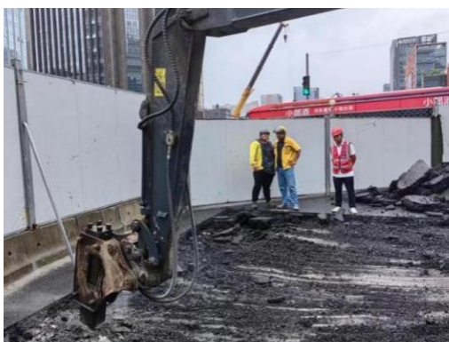
图6 加固区沟槽开挖
