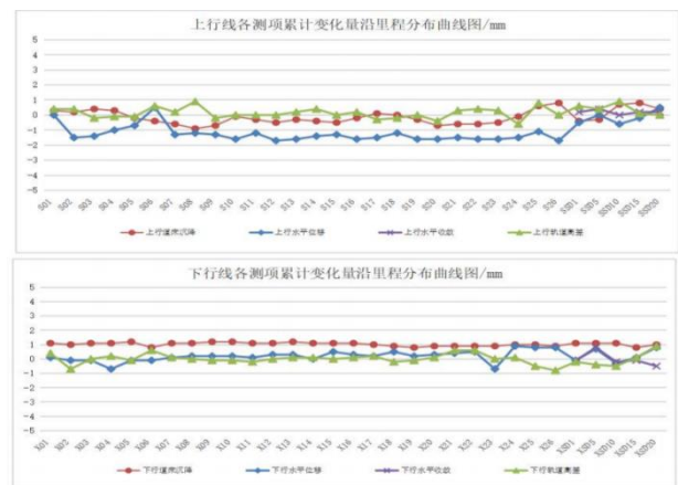
图 13 隧道、车站各测项变化图
