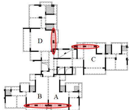
图 3 3#楼结构平面布置图
