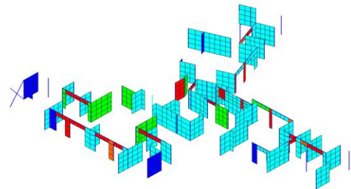
图 12 5#楼构件损伤分布示意图
