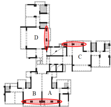
图 2 2#楼结构平面布置图
