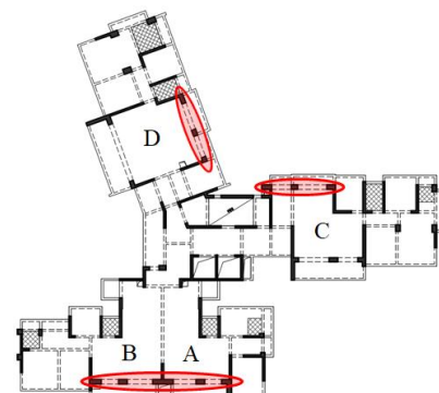
图 4 5#楼结构平面布置图
