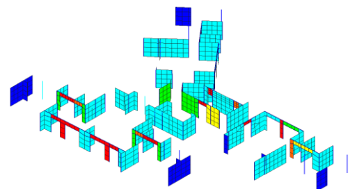
图 13 6#楼构件损伤分布示意图
