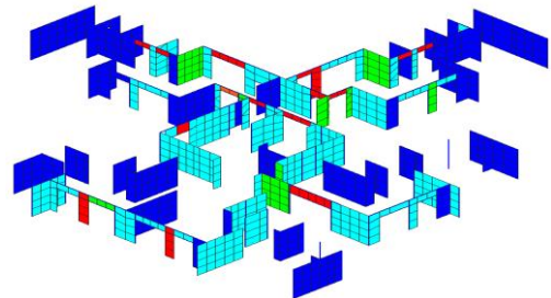
图 9 1#楼构件损伤分布示意图
