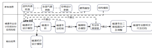
图 4 暖通专业设计阶段 BIM 应用流程
