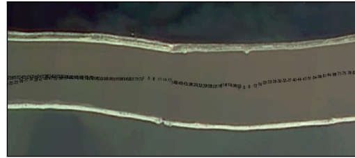
图5 养殖塘测线布设方案
