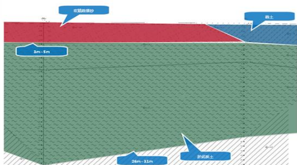
图 1 典型钻孔断面示意图
