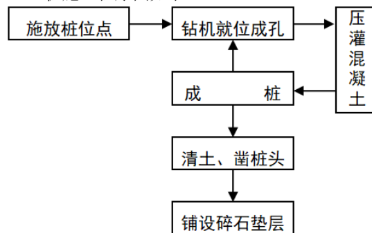
图 1 CFG 桩施工程序图
