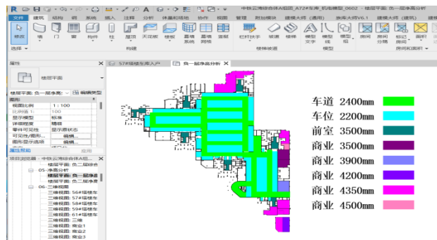
图 6 地库净高分析
