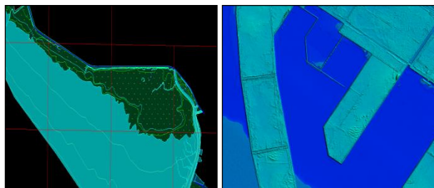
图 6 部分沿海滩涂 DEM 成果 图 7 部分沿海滩涂 DLG 成果
