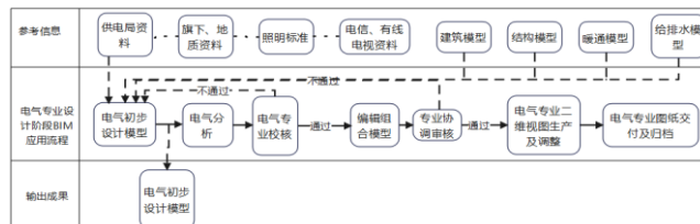
图 5 电气专业设计阶段 BIM 应用流程
