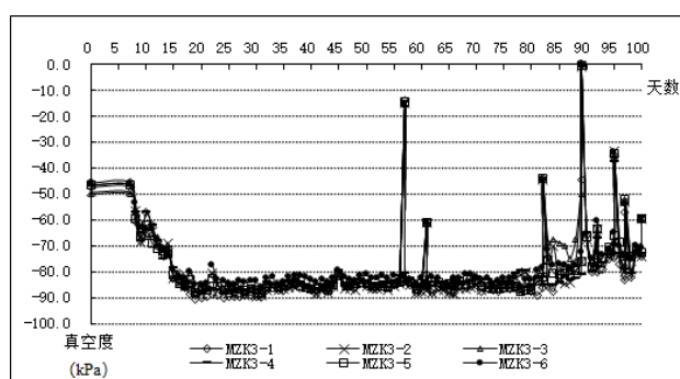
图 2 三区膜下真空度变化过程曲线
