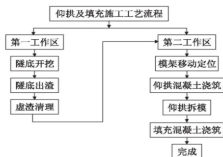
图2 隧道围岩的一种施工工艺流程图
