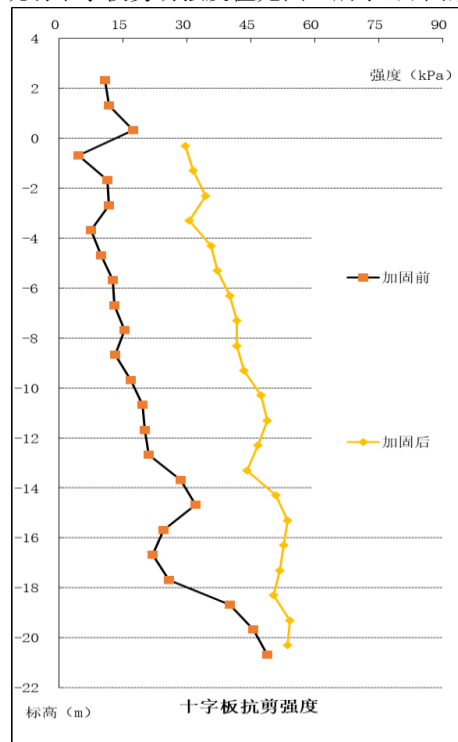
图3 加固前后十字板剪切强度值
