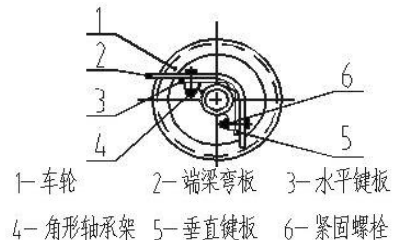
图10 车轮组
