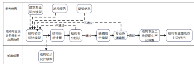
图 2 结构专业设计阶段 BIM 应用流程
