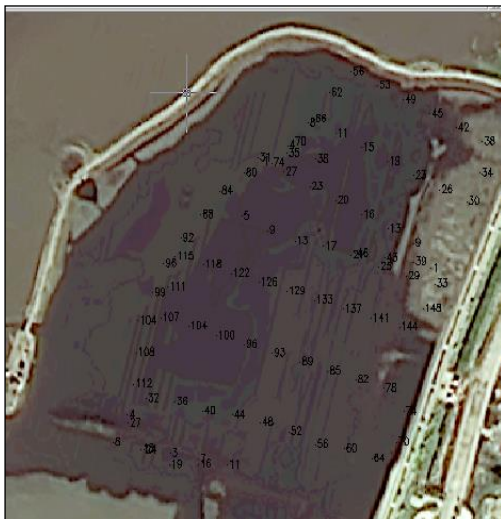
图3 宽河流域测线布设方案
