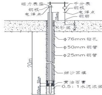
图1 千分表安装示意图
