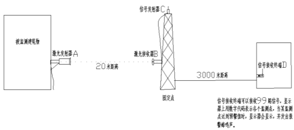
图2 抬动监测及中控预警系统安装示意图
