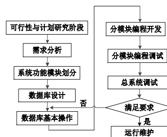
图 1 软件系统开发的流程图
