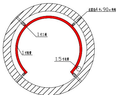
图4 泥浆管路布置示意图
