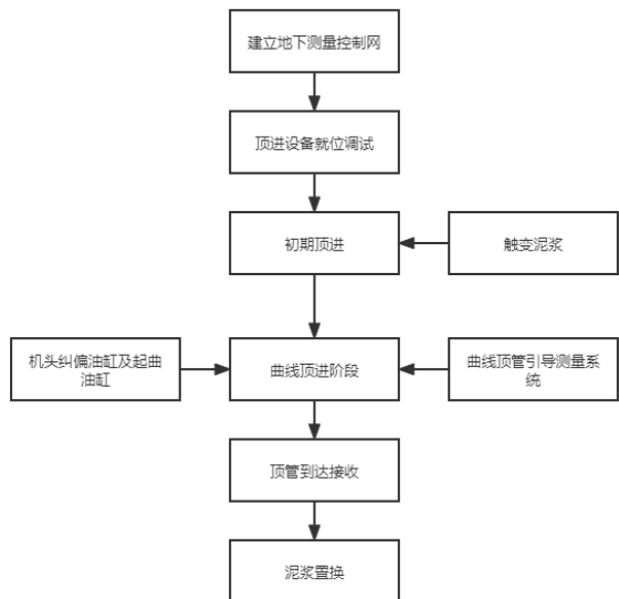
图1 工艺流程图
