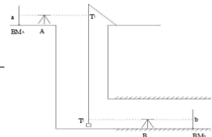
图2 双井定向测量示意图 图3 竖井高程导入测量示意图
