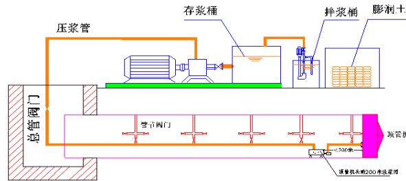
图5 压浆示意图
