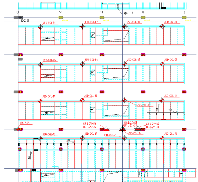
图2 承轨层部分测点安装平面图
