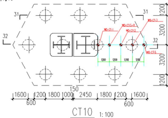
图1 桩基承台温度测点布置
