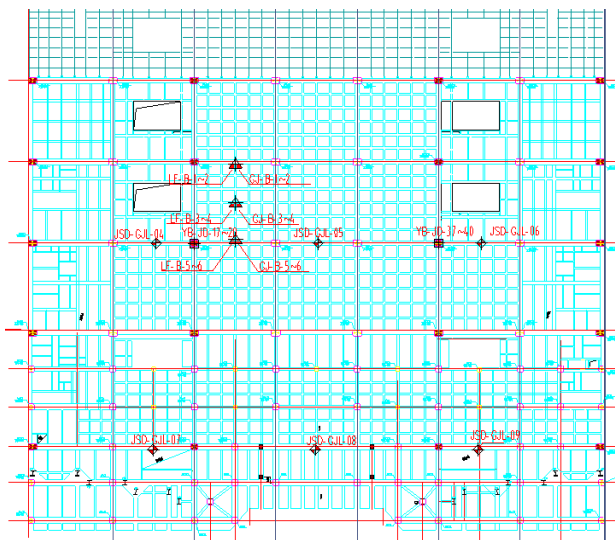
图3 高架层部分测点安装平面图
