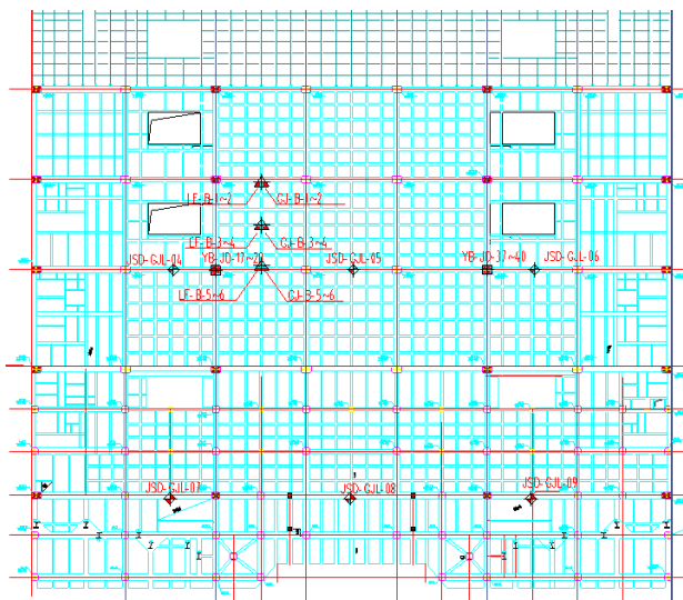
图4 主站房屋盖部分测点安装平面图
