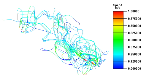
图8 东侧二层鼓型风口流线图
