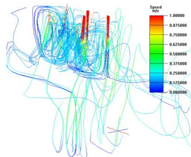
图11 三层典型鼓型风口流线图
