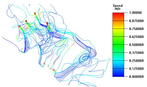
图4 一层气流组织典型条形风口流线图
