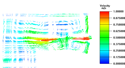
图6 东侧二层鼓型风口矢量图
