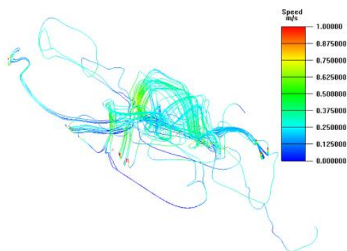
图7 二层典型百叶风口流线图
