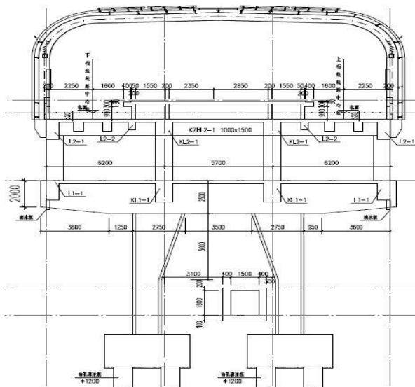
图5 车站横断面图
