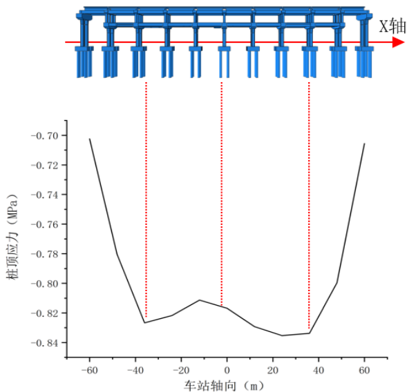
图1 桩基础竖向应力沿车站纵向分布
