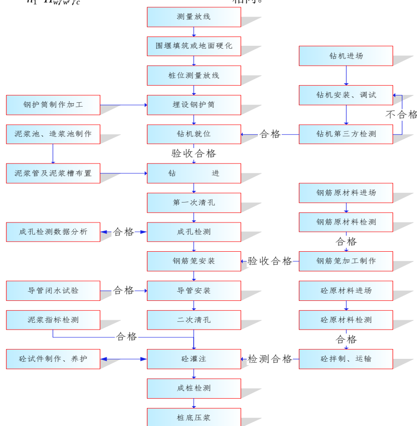
图3 桩基施工工艺流程图
