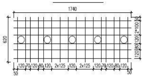
图4 盖梁钢束布置示意图
