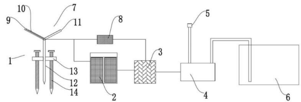
图 1 光伏扬水灌溉系统结构图
