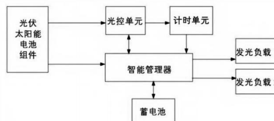
图 2 太阳能 LED 路灯智能管理系统结构示意图
